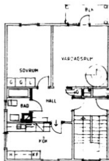
PLAN 2 BOTTENVÅNING
